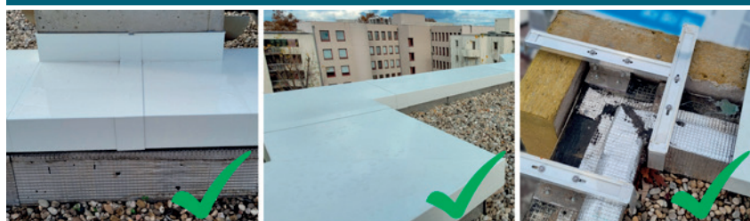
Couvernet ITE sur console TH pour acrotère isolé pièces spéciales préfabriquées en usine
